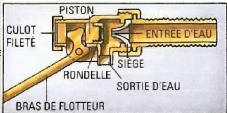
Chasse d'eau à alimentation par le dessous avec robinet flotteur silencieux
